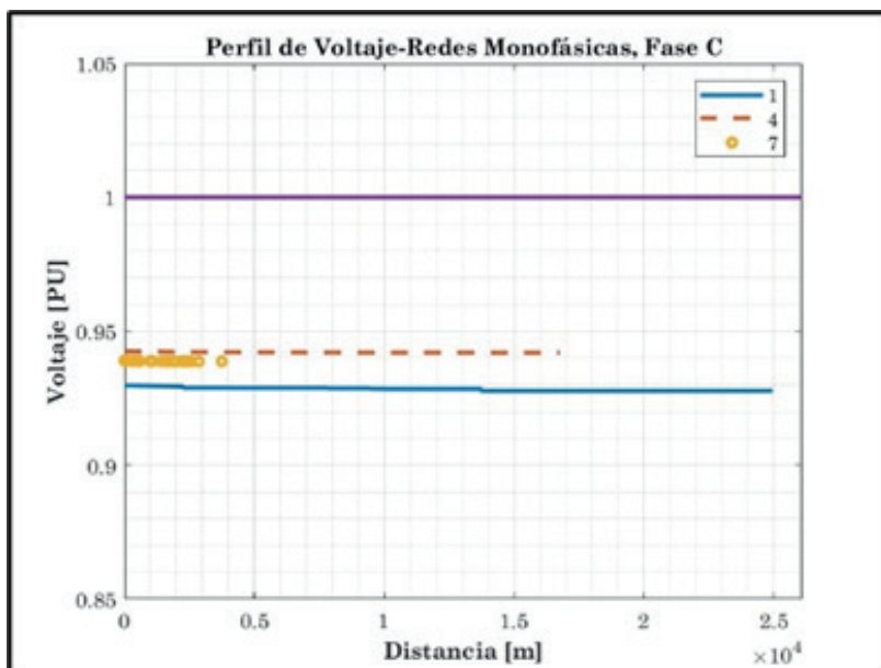
Figura 26. Perfil de voltaje, redes monofásicas conectadas a la fase C.
