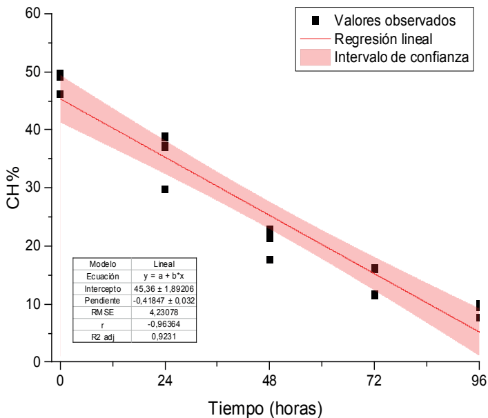
Figura 10. Modelo lineal de la curva de secado de la madera ajustado a los valores de CH% observado durante el tiempo de secado. RMSE: Raíz del error cuadrático medio o desviación estándar de los residuos; r: coeficiente de correlación; R 2 adj: Coeficiente de determinación ajustado.
