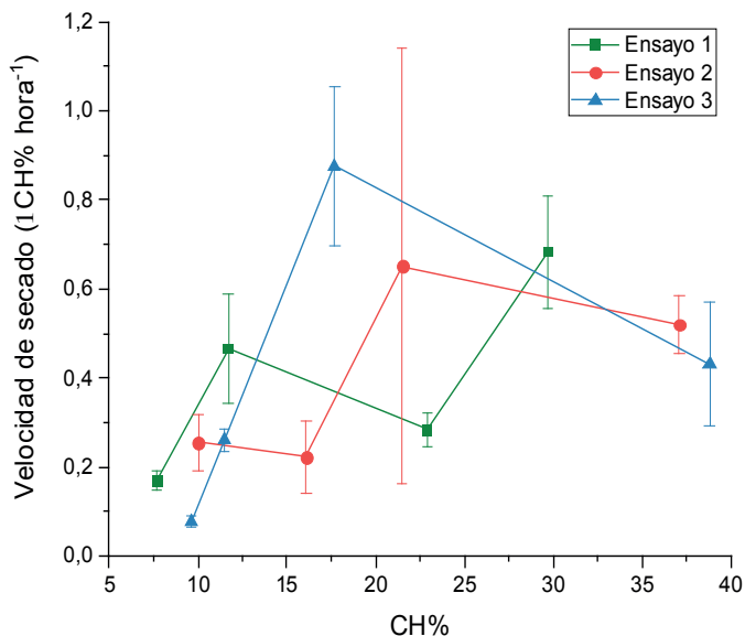
Figura 12. Curva de velocidad de secado ( \Delta\text{CH}\% hora -1 ) por ensayo. Expresa la cantidad de humedad evaporada en la madera ( \Delta\text{CH}\% ) en una hora de secado a diferentes CH% de humedad. El secado es más lento cuanto menor es el CH% de la madera
