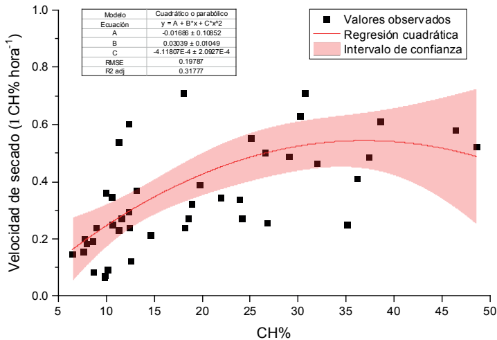
Figura 14. Modelo no lineal (cuadrático o parabólico) de la curva de velocidad de secado. RMSE: Raíz del error cuadrático medio o desviación estándar de los residuos; R 2 adj: Coeficiente de determinación ajustado.
