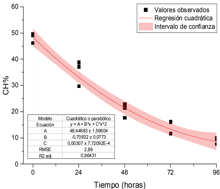
Figura 11. Modelo no lineal (cuadrático o parabólico) de la curva de secado de la madera ajustado a los valores de CH% observado durante el tiempo de secado. RMSE: Raíz del error cuadrático medio ó desviación estándar de los residuos; R 2 adj: Coeficiente de determinación ajustado.
