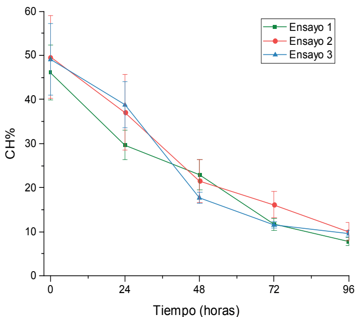
Figura 9. Curva de secado de la madera, que representa la evolución del contenido de humedad de la madera (CH) con el tiempo de secado, por ensayo. Las barras verticales indican la desviación estándar de la media.
