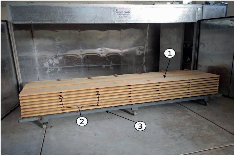
Figura 7. Elementos del paquete (1. Madera cortada, 2. Espaciadores, 3. Parrilla)
