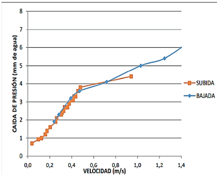
Figura 01. Curvas de caída de presión contra velocidad para un diámetro de 13.5 cm y altura de 25 cm.
