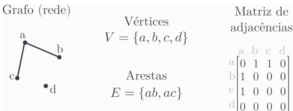
Figura 3 Diferentes formas de representação de um grafo. Sua representação imagética como rede (à esquerda), sua representação algébrica, como conjuntos de vértices e de arestas, e sua representação por uma matriz de adjacências
