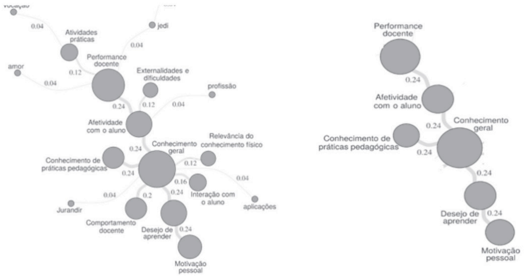
Figura 3 Exemplo de decomposição seguindo a propriedade dual
