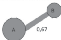
Figura 2 Detalhamento da construção de uma rede de similaridades entre pares de termos evocados.
