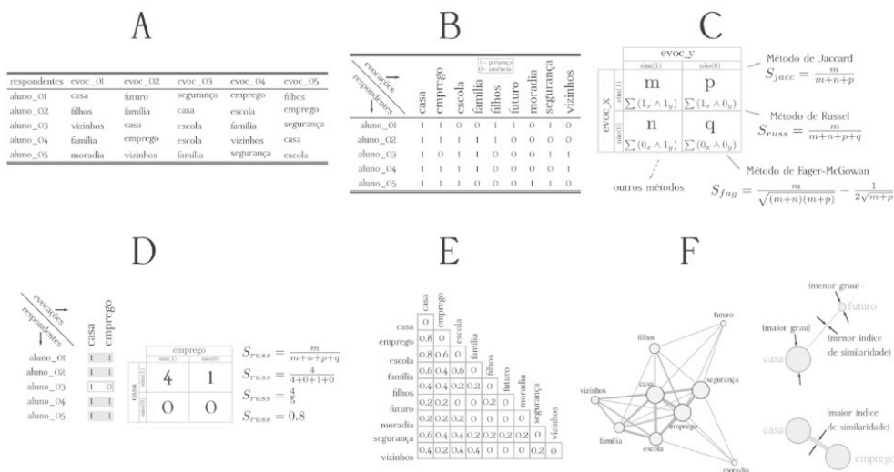
Figura 5 Passo a passo da construção de uma rede hipotética de similaridades, a partir de um conjunto de cinco palavras evocadas por cada um de cinco sujeitos de pesquisa, utilizando o algoritmo de similaridade de Russel
