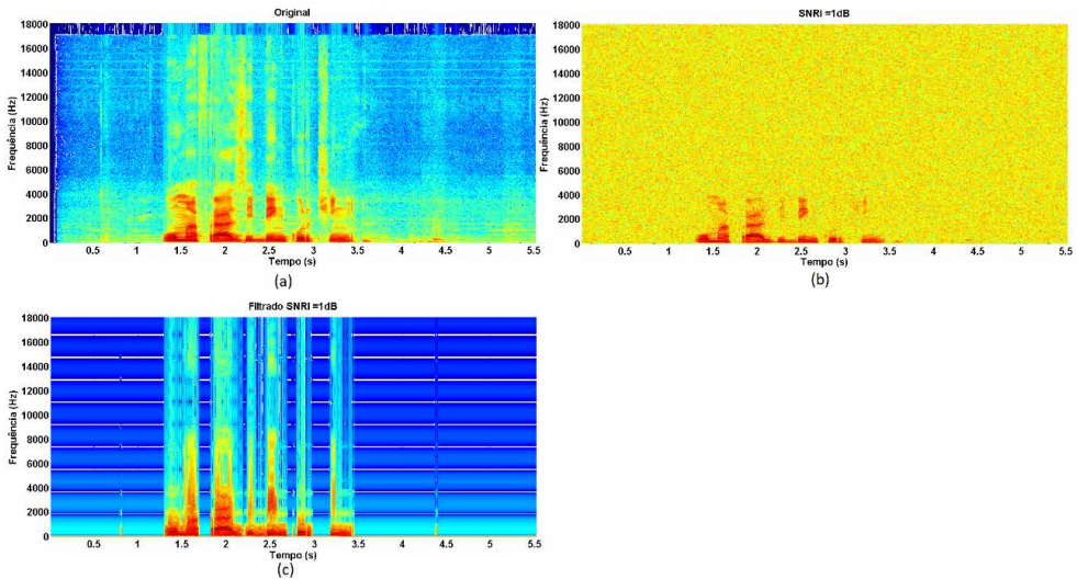
Figura 6. (a) Espectrograma do sinal original; (b) espectrograma do sinal com ruído aditivo e SNR_i(\text{dB}) = 1 ; (c) espectrograma do sinal ( SNR_i = 1\text{dB} ) após a filtragem com o método limiar Hard-Thresholding .
