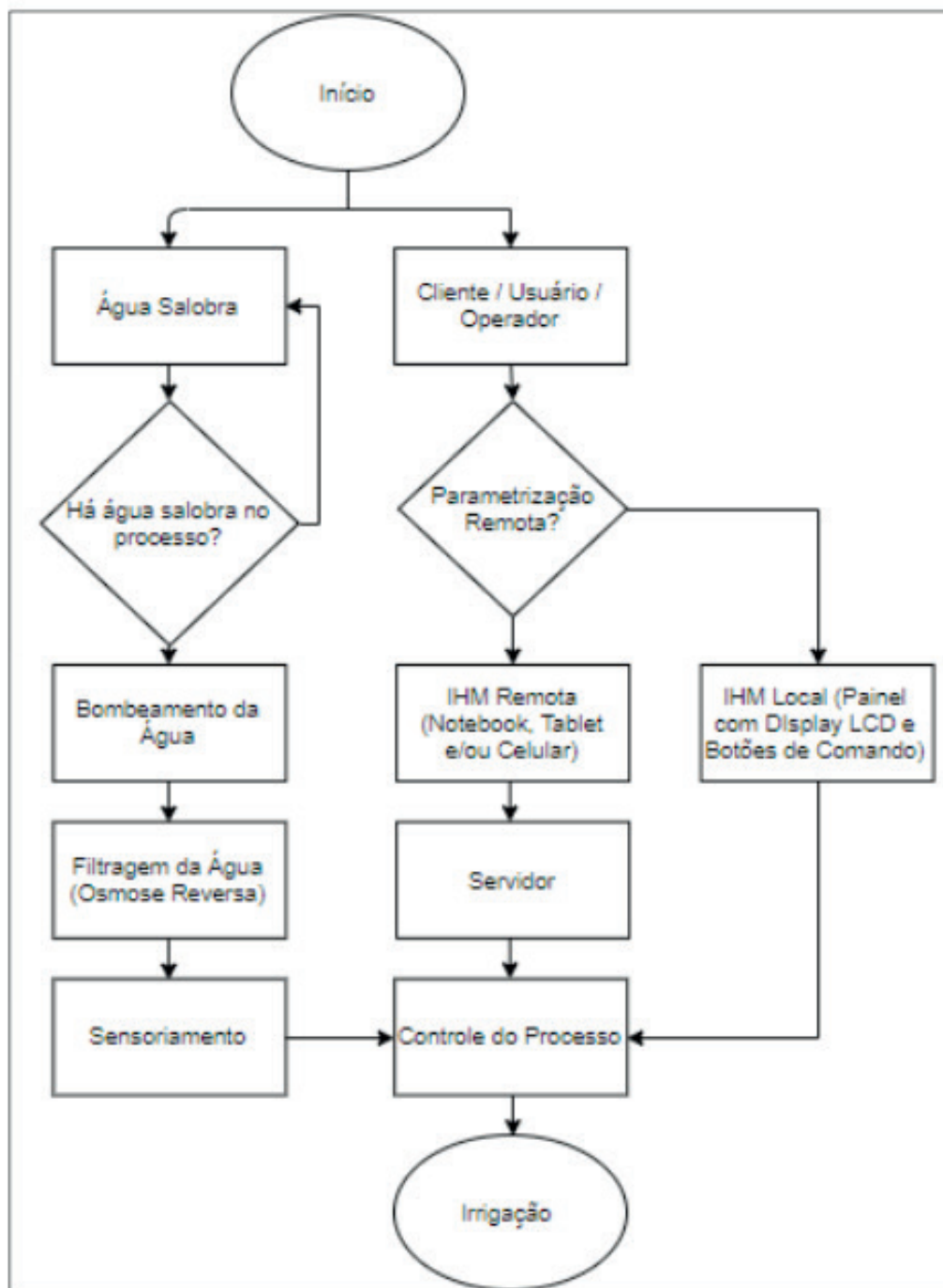
Figura 13 – Fluxograma do processo
