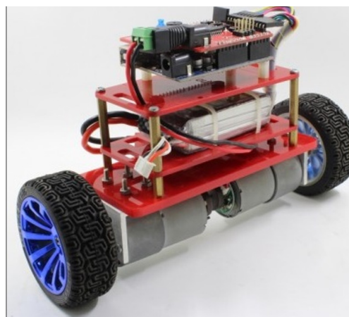
Figura 1 - Robô móvel de duas rodas.
