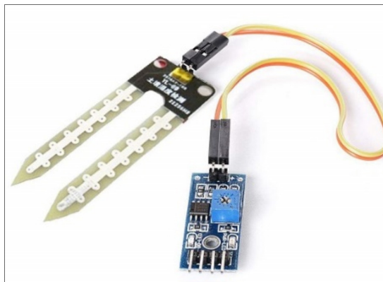
Figura 8 - Sensor de Umidade YL-69
