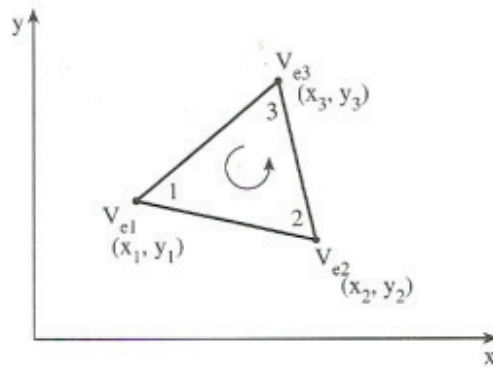
Fig. 3. Elemento triangular típico; nó local numerado 1 – 2 - 3 deve proceder o sentido anti-horário conforme indicado pela seta. [9]
