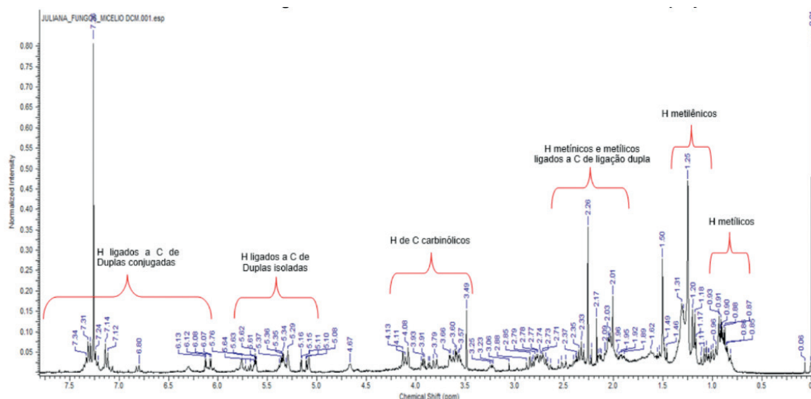
Figura 1: Espectro de Ressonância Magnética Nuclear de ^1\text{H} (300 MHz, \text{CDCl}_3 ) do extrato diclorometânico do micélio do fungo endófito Dm SB 43 de Duroia macrophylla .
