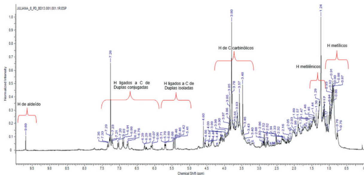
Figura 3: Espectro de Ressonância Magnética Nuclear de ^1\text{H} (300 MHz, \text{DMSO-}d_6 ) da fase diclorometânica do caldo metabólico do fungo endofítico Dm BDA 13 de Duroia macrophylla .
