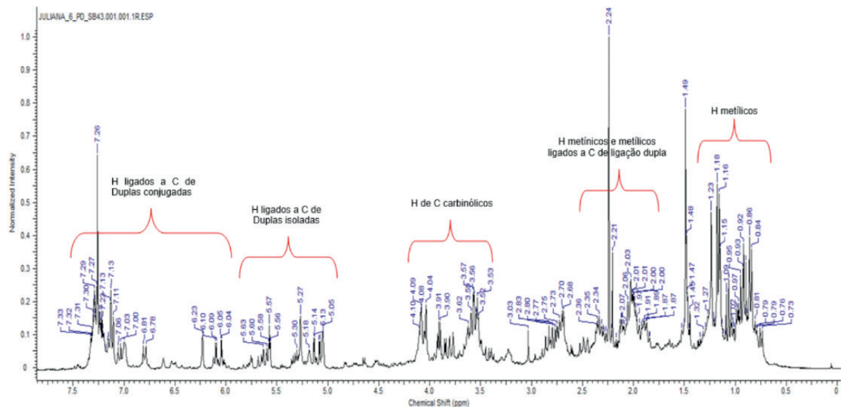
Figura 2: Espectro de Ressonância Magnética Nuclear de ^1\text{H} (300 MHz, \text{DMSO-}d_6 ) da fase diclorometânica do líquido metabólico do fungo endofítico Dm SB 43 de Duroia macrophylla .
