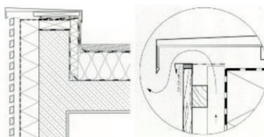
DET 10: Corte.
