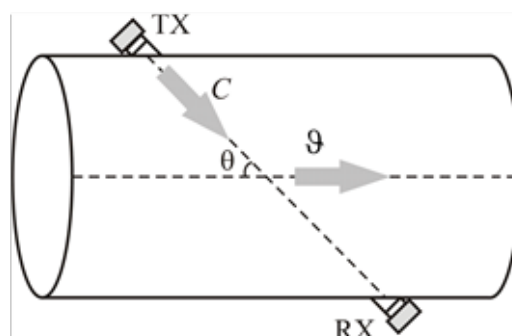
Figura 2. Configuração dos sensores para medição
