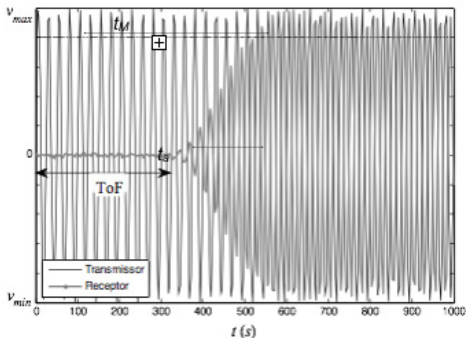
Figura 5. Medição do ToF utilizando a técnica de Detecção de Limiar (TH).
