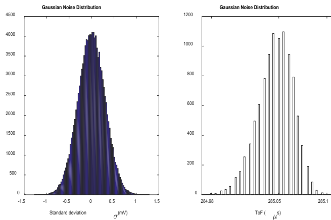
Figure 12. FDP do ToF usando ruído Gaussiano com \sigma=0.3 mV.
