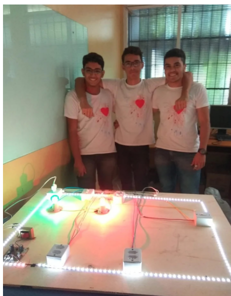
Figura 4: Projeto de um ambiente residencial construído pelos alunos Autoria própria
