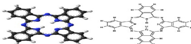
Fig.01- Estrutura molecular da ftalocianina de base livre
