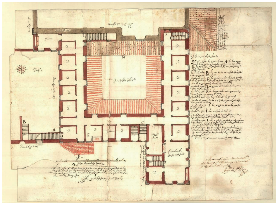
Fig. 15. S. a., planta do Convento dos Remédios, 1719, Évora. Fonte: Câmara Municipal de Évora.
