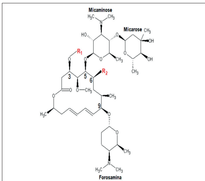
Figura 4: Estrutura química dos principais componentes da espiramicina e suas substâncias relacionadas. Fórmula molecular : C_{43}H_{74}N_2O_{14} .
