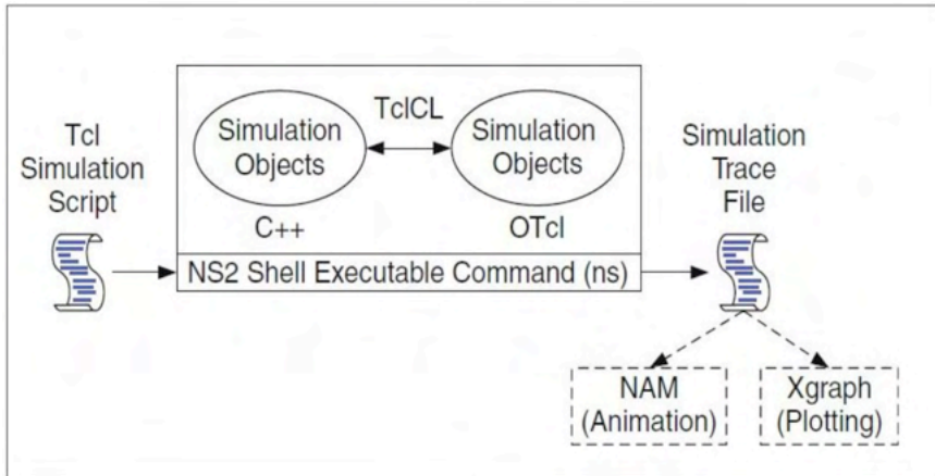
Figura 9. Arquitetura do NS2 [9].
