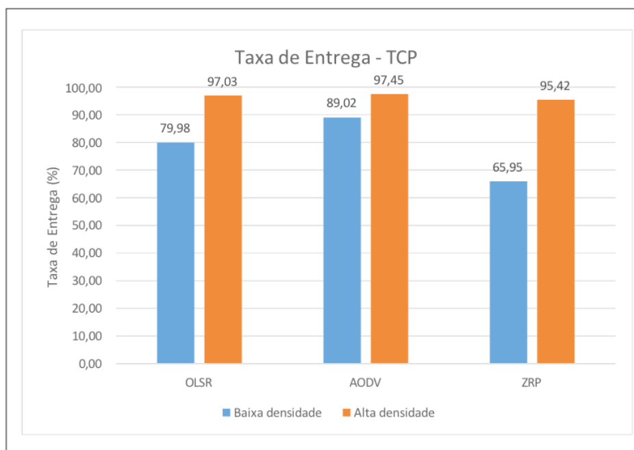
Figura 16. Taxa de entrega TCP
