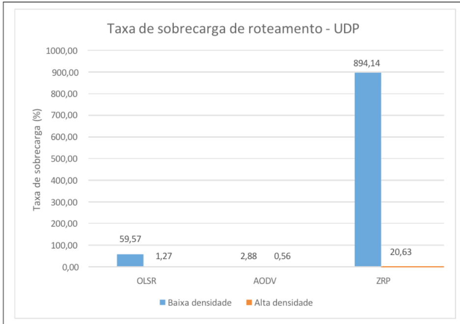
Figura 21. Taxa de sobrecarga UDP
