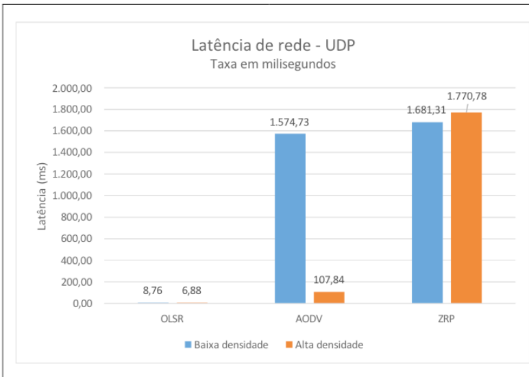
Figura 13. Latência UDP
