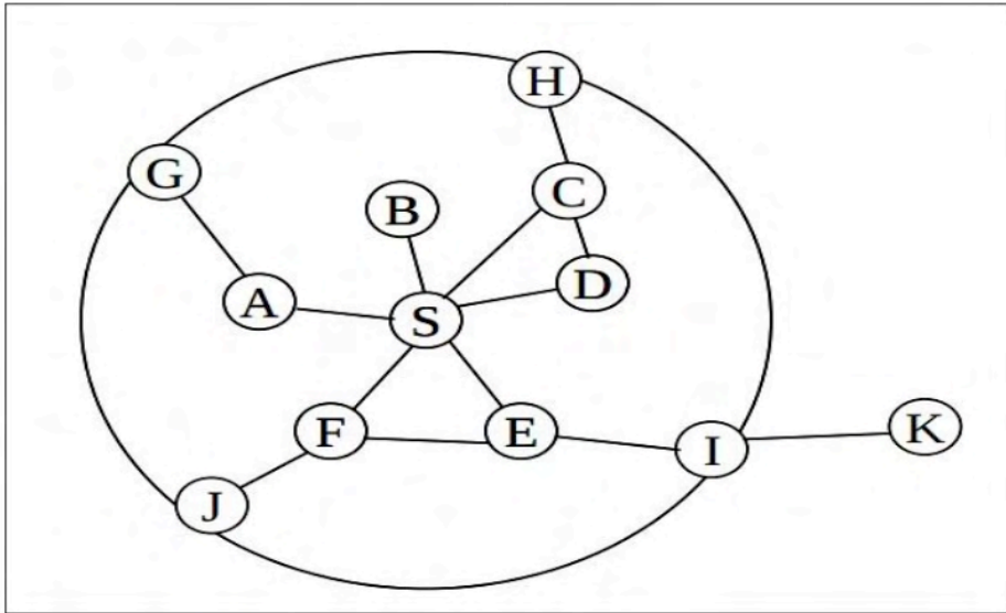
Figura 6. Exemplo do mecanismo Zone Radius ZRP [6].
