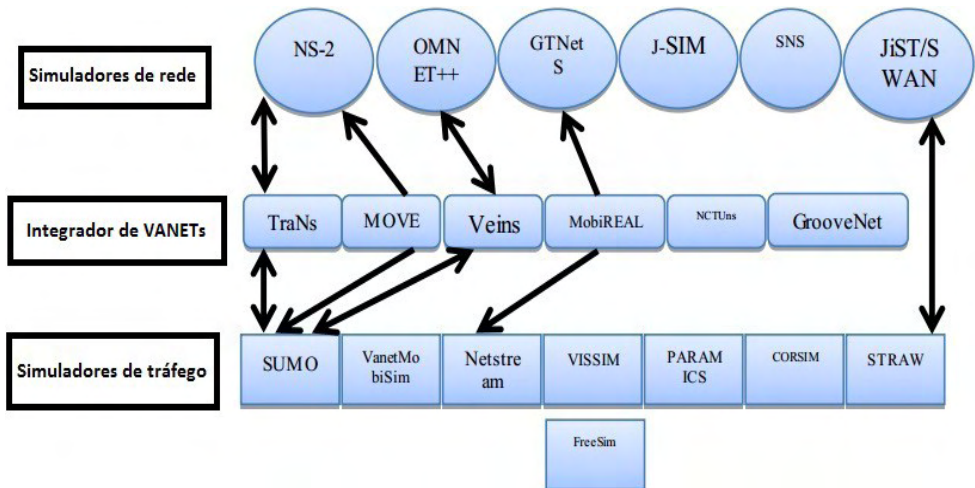
Figura 8. Classificação de simuladores veiculares. Adaptado de [8]
