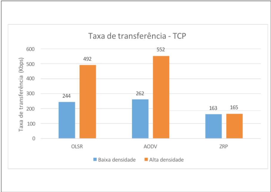
Figura 24. Taxa de transferência TCP
