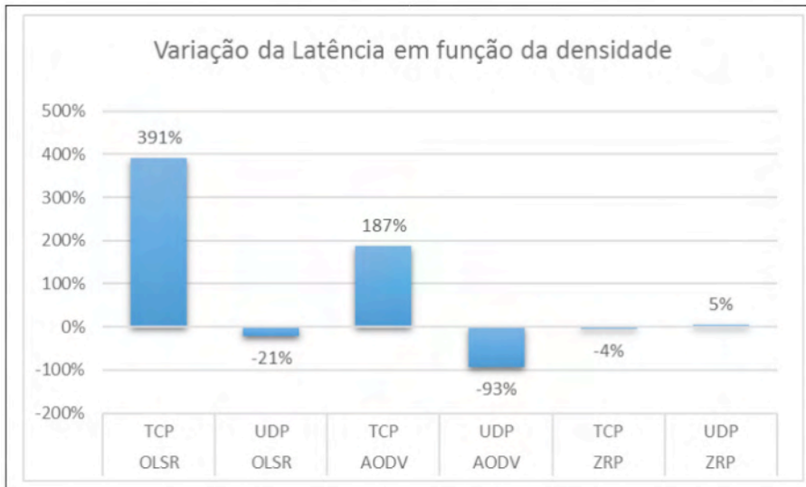
Figura 14. Variação da Latência em função da densidade
