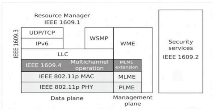
Figura 3. Arquitetura de protocolos IEEE 1609 e IEEE 802.11p [3].
