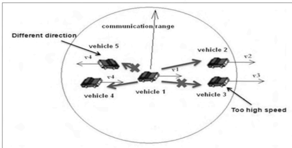
Figura 5. Exemplo de seleção de vizinhança com AODV [5].
