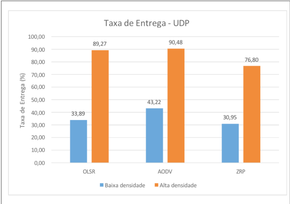
Figura 17. Taxa de entrega UDP
