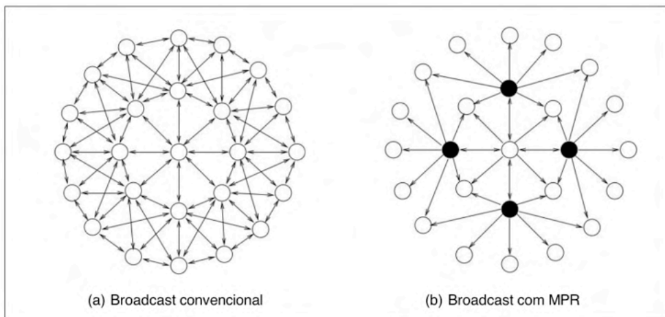
Figura 4. Formato de broadcast OLSR [4]
