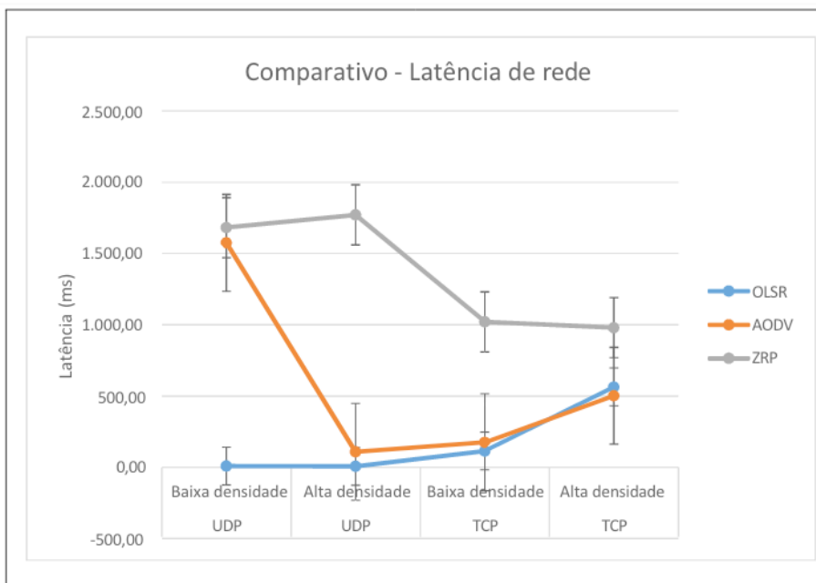
Figura 15. Comparativo da latência em função das densidades
