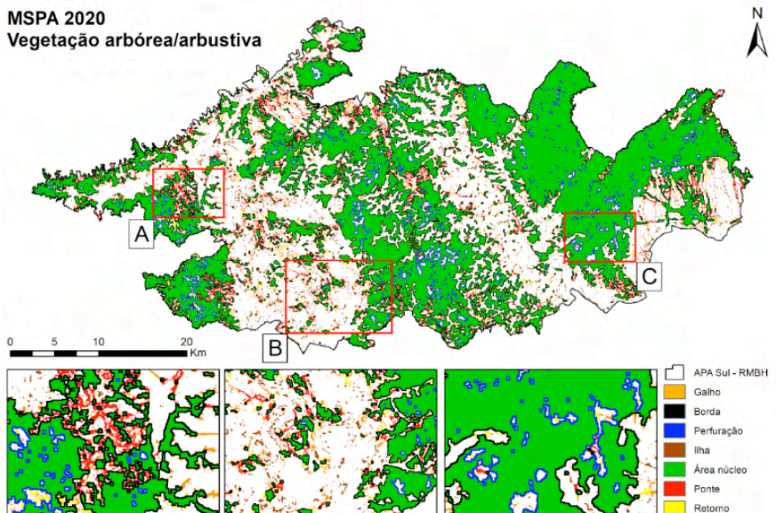
Figura 7: MSPA do ano inicial (1985) e ano final (2020) da série histórica analisada.
