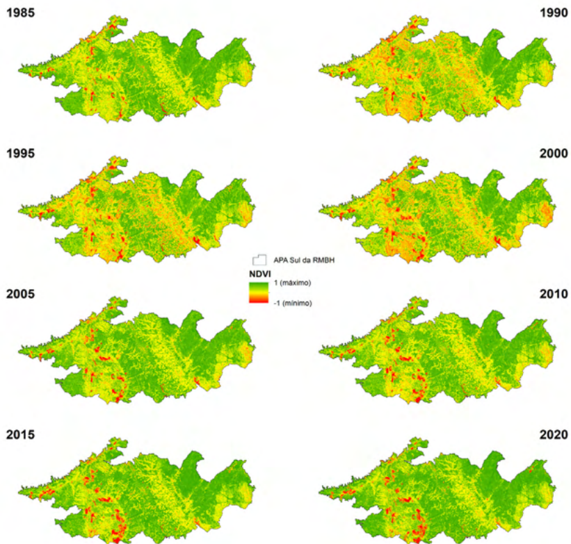
Figura 5: NDVI obtido a partir de script implementado no Google Earth Engine.
