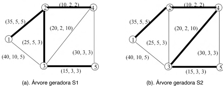
Figura 7. Conjunto final das árvores geradoras mínimas fuzzy – Instância 1.
