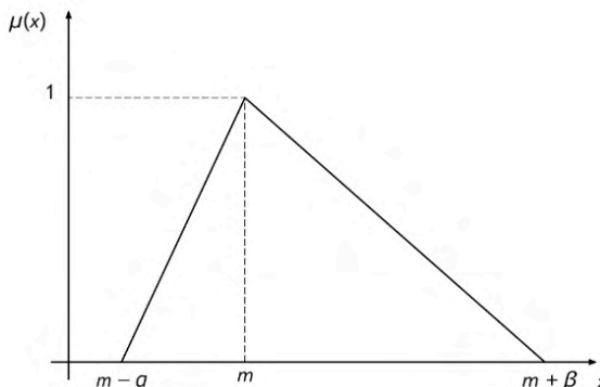
Figura 1. Exemplo de uma função de pertinência triangular.
