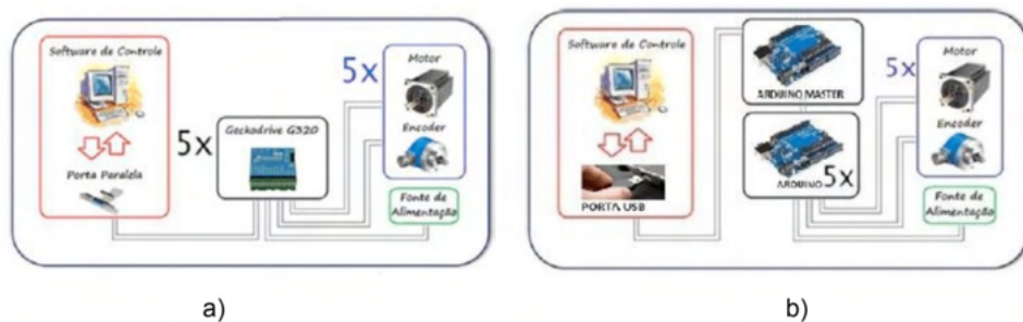
Figura 1: Arquiteturas de controle do Manipulador ASEA IRB6.
