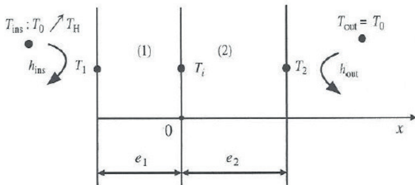
Figura 1: Apresentação do problema de duas camadas a ser solucionado pelo método Quadrupolo.
