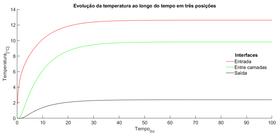
Figura 2: Evolução da temperatura ao longo do tempo nas três posições analisadas.
