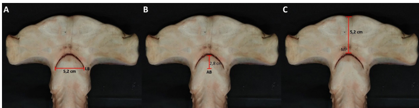
Figura 3. Vista ventral de tubarão-martelo, Sphyrna lewini demonstrando as medidas da boca. (A) Largura da Boca (LB). (B) Altura da Boca e (C) Medida Pré-oral.
