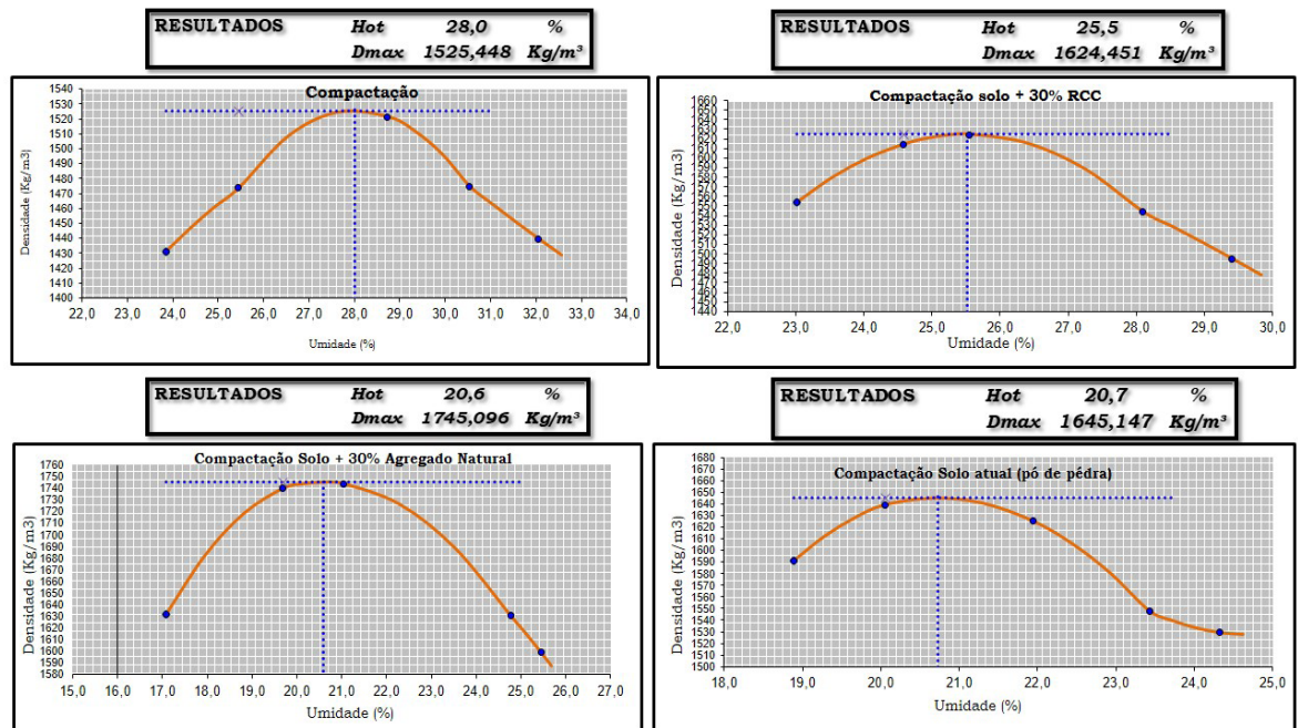
Figura 3: Ensaio de Compactação.
