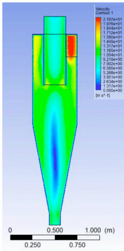
Figura 7. Perfil de velocidade Ciclone 1.
