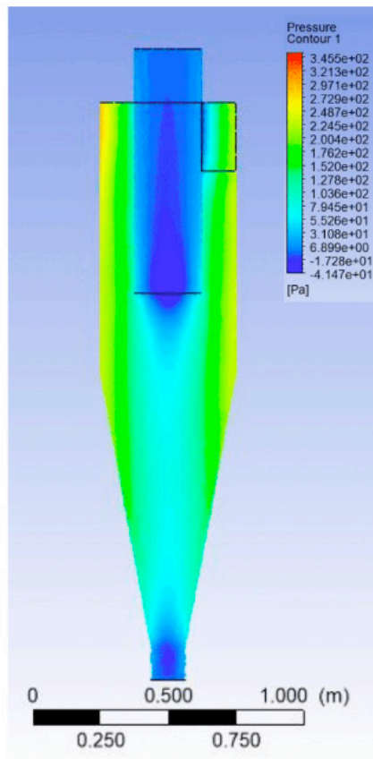
Figura 5. Perfil de pressão Ciclone 2.
