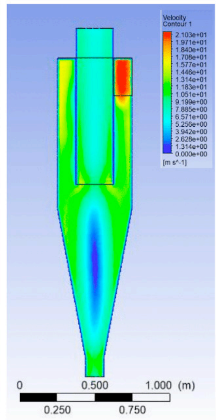
Figura 9. Perfil de velocidade Ciclone 3.
