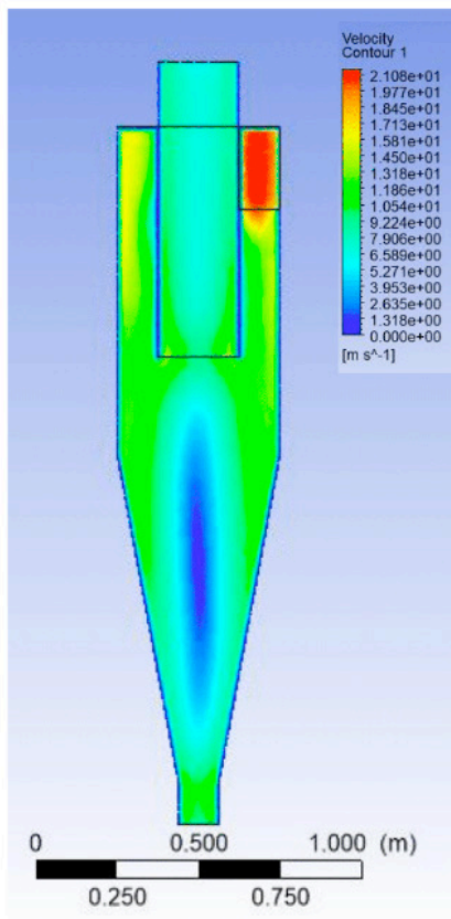
Figura 8. Perfil de velocidade Ciclone 2.
