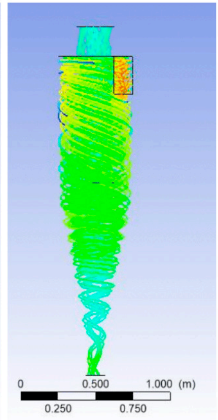
Figura 12. Linhas de fluxo Ciclone 3.
