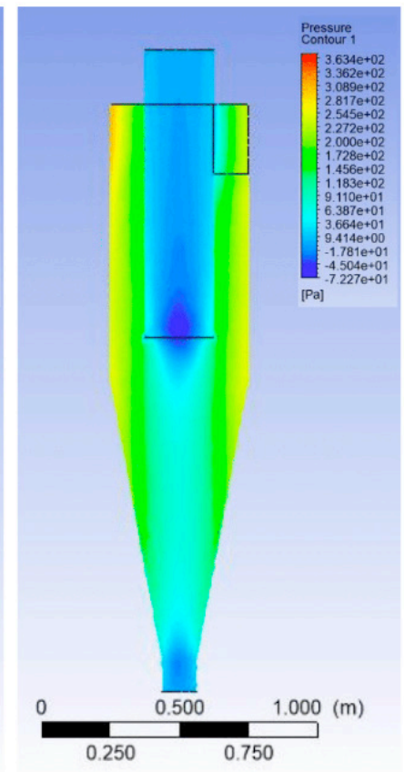
Figura 6. Perfil de pressão Ciclone 3.
