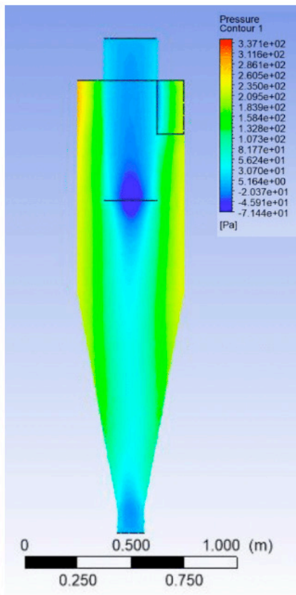
Figura 4. Perfil de pressão Ciclone 1.
