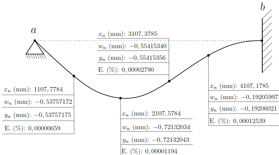
Figura 2 - Deflexão no eixo longitudinal da viga apoiada-engastada.
