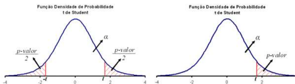
Figura 2- Função Densidade de Probabilidade para t de Student. Fonte: Autores, 2016
