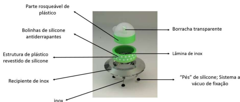
FIGURA 8 – Detalhamento da modelagem tridimensional no 3ds MAX® da Autodesk. Fonte: Autores (2016).
