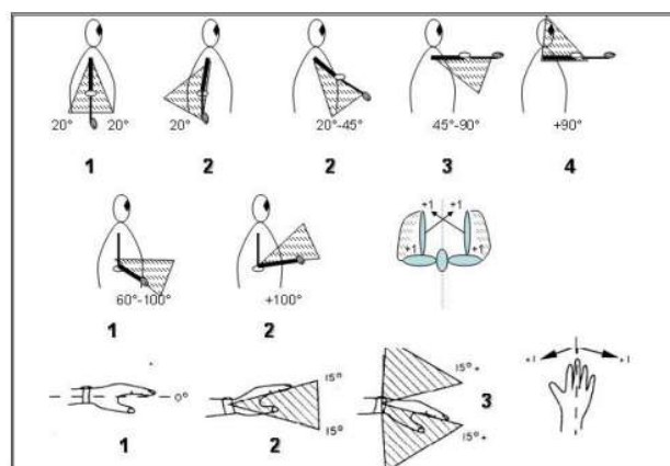
FIGURA 2 – Diagrama das posturas adotadas para o grupo A. Fonte: McAtamney e Corlett (1993), adaptado.
