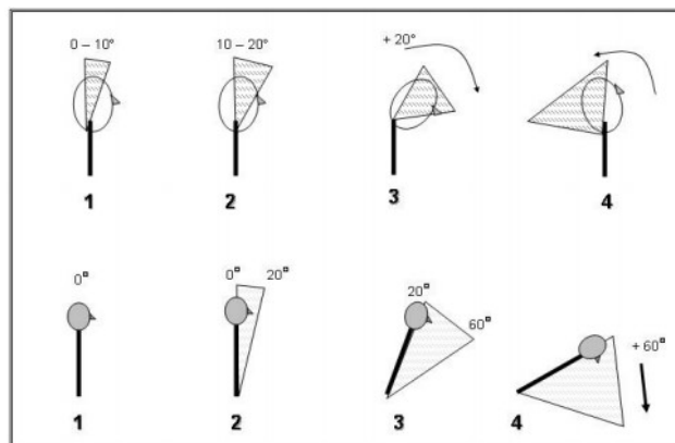
Figura 3 – Diagrama de Posturas adotadas para o Grupo B. Fonte: McAtamney e Corlett (1993), adaptado.
