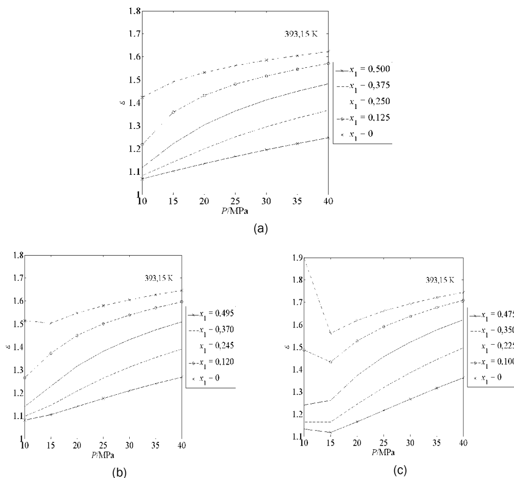
Figura 2 – Perfil da constante dielétrica para: (a) CO 2 (1) + Metano (2) + Propano (3); (b) CO 2 (1) + Metano (2) + Propano (3) + H 2 O (4) (1%); (c) CO 2 (1) + Metano (2) + Propano (3) + H 2 O (4) (5%).
