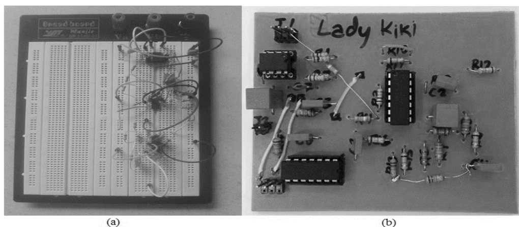
Figura 6 – Protótipo de eletromiógrafo: (a) Montado em uma protoboard; (b) Montado em Placa de Circuito Impresso.
