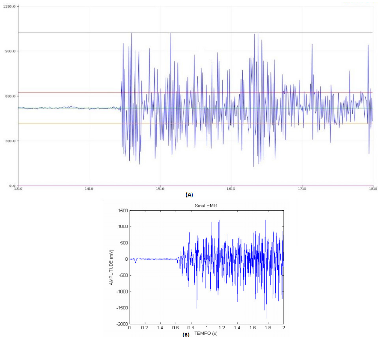
Figura 9 – (a) Visualização dos sinais de EMG digitalizados através do Arduíno (b) EMG na literatura. Fonte: (MARCHETTI; DUARTE, 2006, p. 12).
