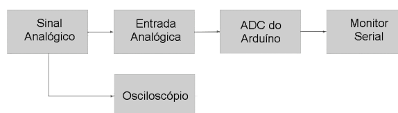
Figura 4 – Diagrama de blocos do algoritmo para visualizar os sinais de EMG.
