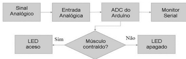
Figura 5 – Diagrama de Blocos do algoritmo desenvolvido para detecção de músculo contraído.
