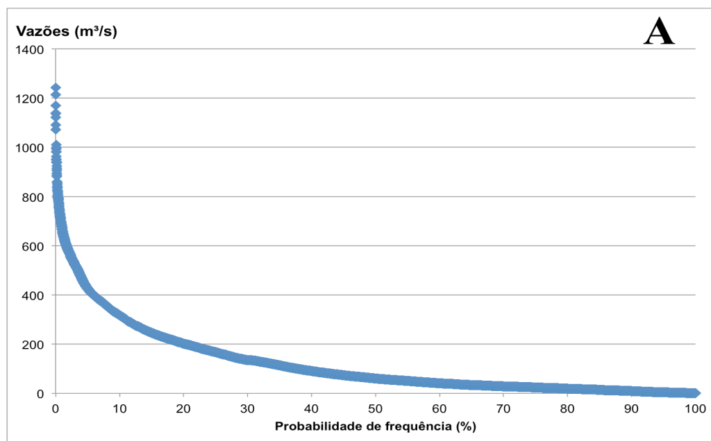
Gráfico 1 – Dados de vazão do rio Maicuru para avaliação da vazão de referência.
