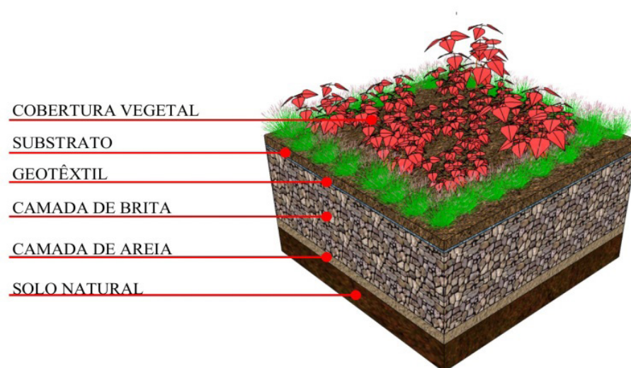
Figura 6. Exemplo de telhado verde. MELO, 2011.
