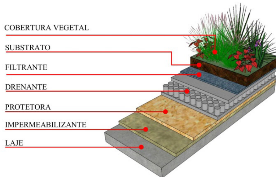
Figura 6. Exemplo de telhado verde. MELO, 2011.
