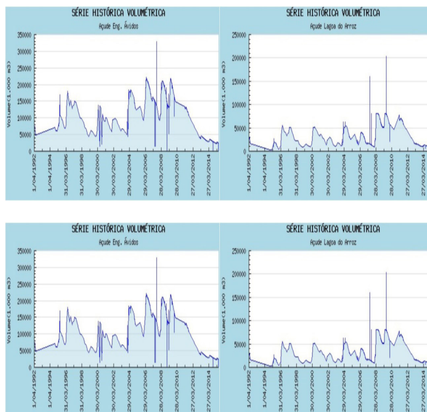
Figura 2. Séries históricas volumétricas dos açudes Engenheiros Ávidos e Lagoa do Arroz, respectivamente, em Cajazeiras (1992 – 2015). DNOCS, 2016.
