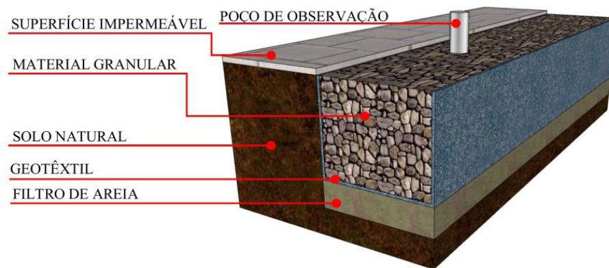
Figura 5. Exemplo de trincheira de infiltração. MELO, 2011.
