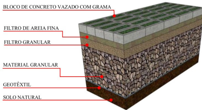
Figura 4. Exemplo de pavimento permeável de blocos de concreto vazados preenchidos com grama. MELO, 2011.
