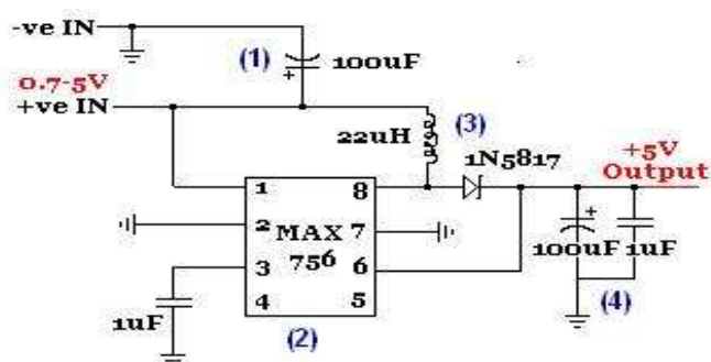
Figura 7 - Circuito Elevador de Tensão
