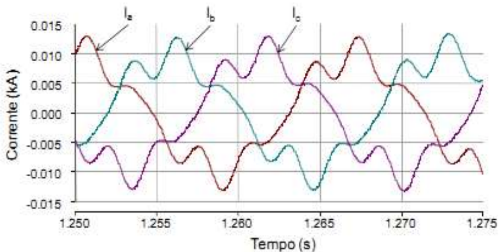
Figura 5 – Corrente do conversor com DSTATCOM
